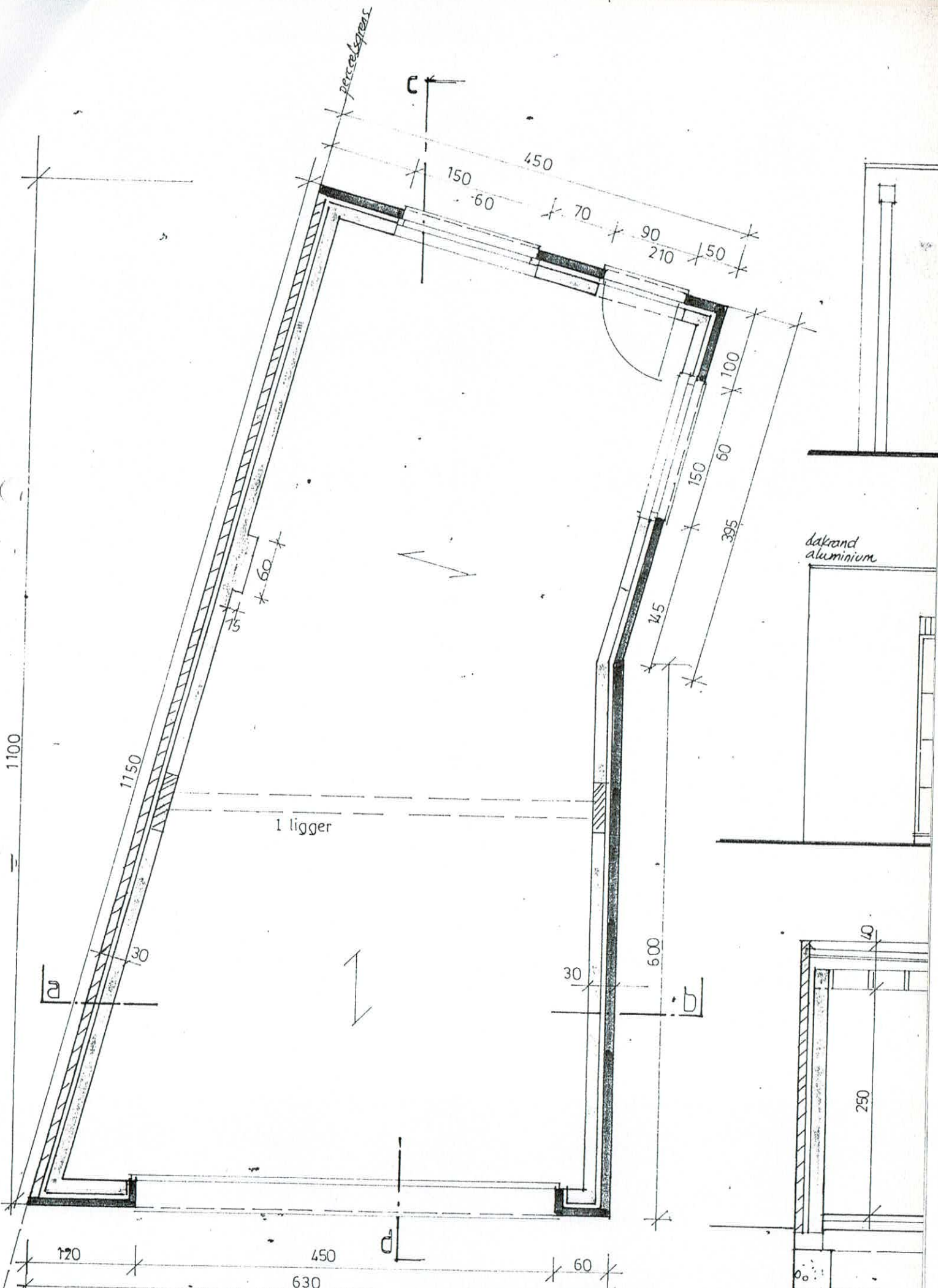
GRONDPLAN
