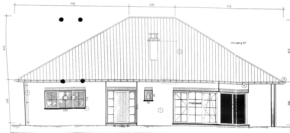
ZIJGEVEL RECHTS
