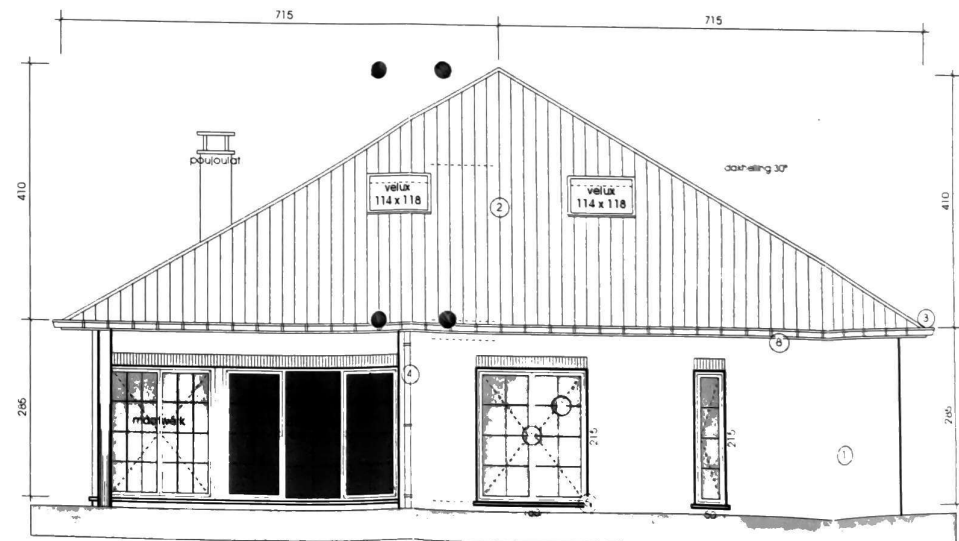
ACHTERGEVEL
