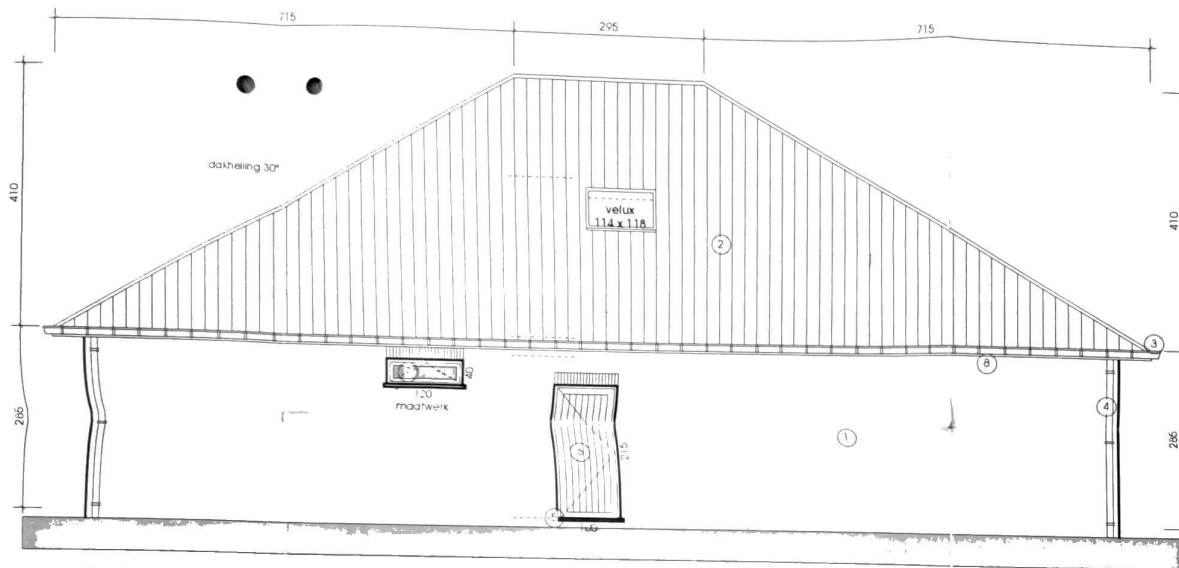
ZIJGEVEL LINKS
